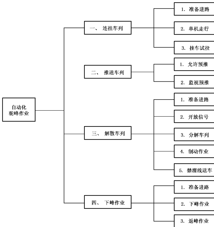
图 1 铁路调车自动化驼峰作业程序图
