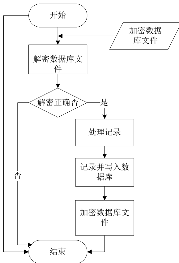
图 3.7 数据库库外加密流程图
