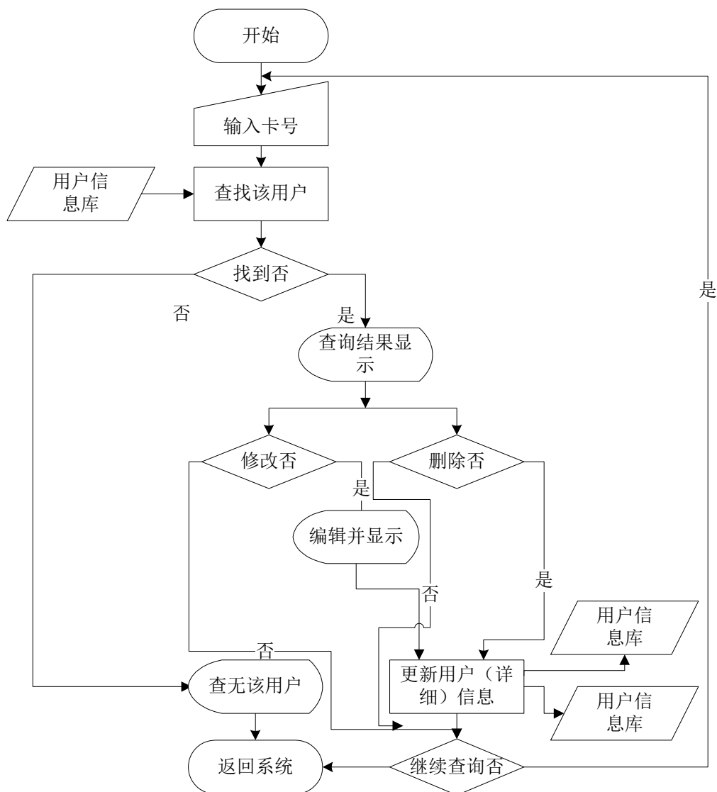
图 3.2 用户档案查询修改模块流程图图
