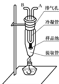
图 1 微型提取器的结构
