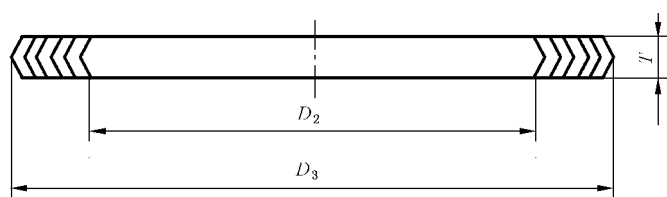
图 1 基本型缠绕式垫片
