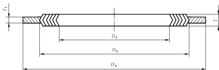
图 3 带定位环型缠绕式垫片
