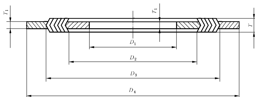
图 4 带内环和定位环型缠绕式垫片
