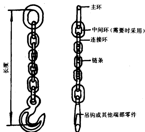
图1 单肢链式吊索
