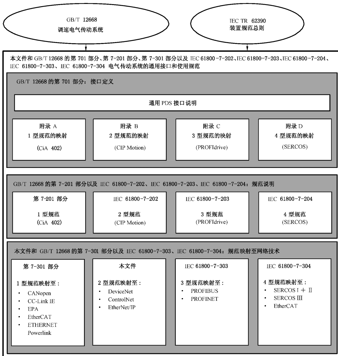
图 1 本文件和 GB/T 12668 的第 701 部分、第 7-201 部分、第 7-301 部分以及 IEC 61800-7-202、IEC 61800-7-203、IEC 61800-7-204、IEC 61800-7-303、IEC 61800-7-304 的结构
