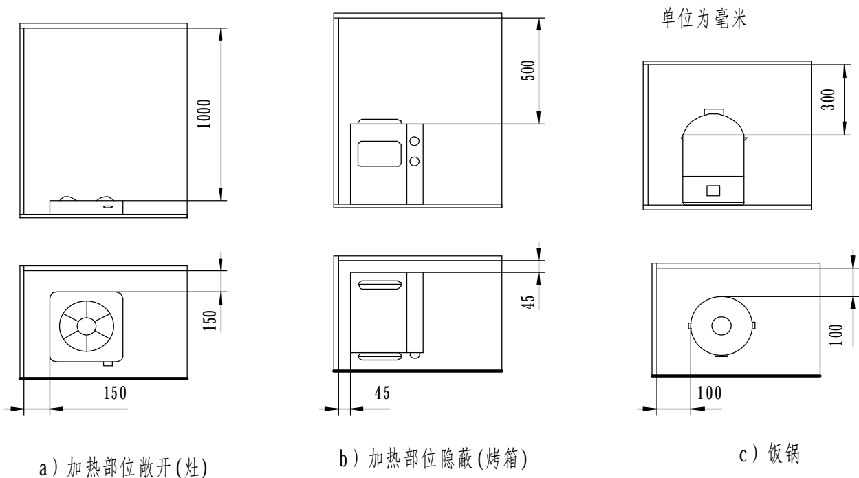
图 9 木壁、木台表面温升试验装置
