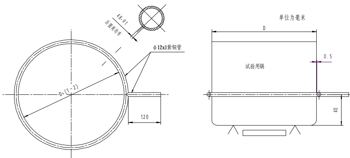
b) 燃气灶烟气取样位置
