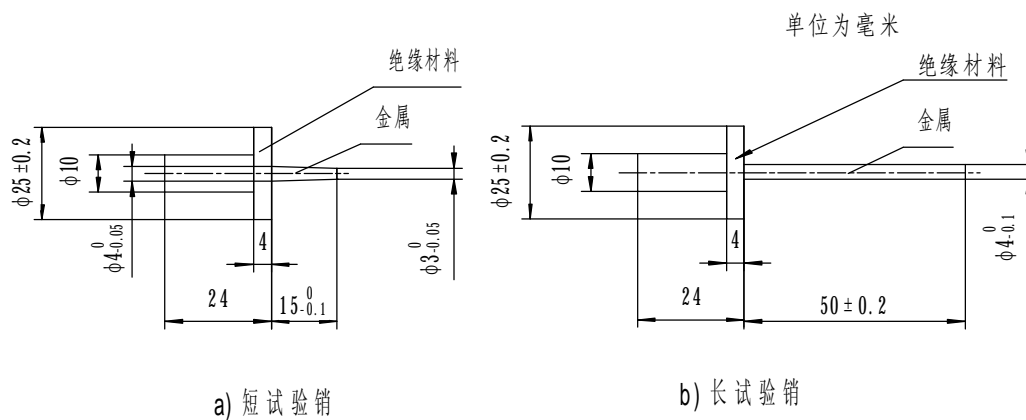
图3 试验销
