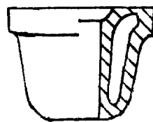
空腔式风口
