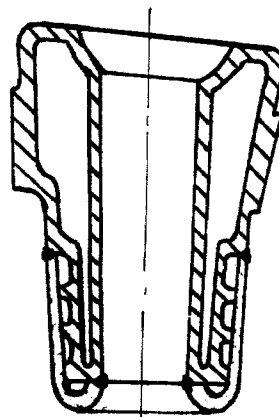
贯流式风口
