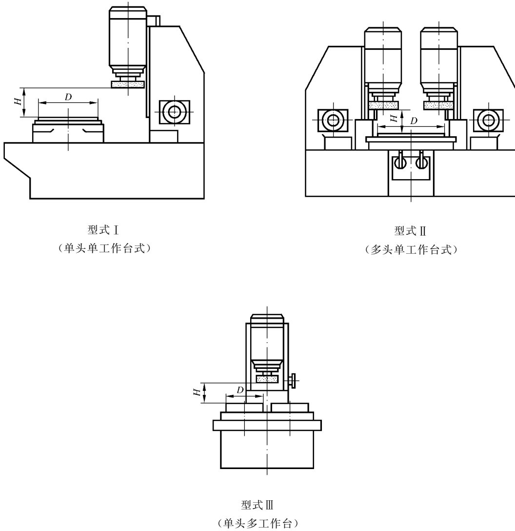
图 1 立轴圆台平面磨床型式
