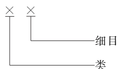
图 1 代码结构图
