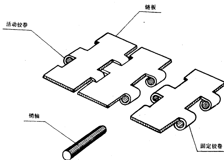
图1 平顶链
