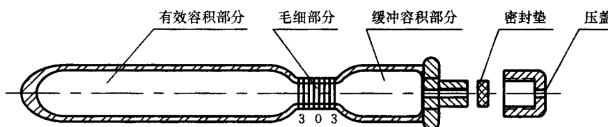
图 1 压力密度瓶示意图
