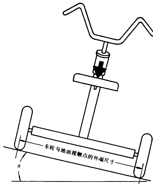
图1 车辆行驶的稳定性的试验
