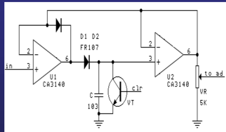
图9 峰值检波电路
