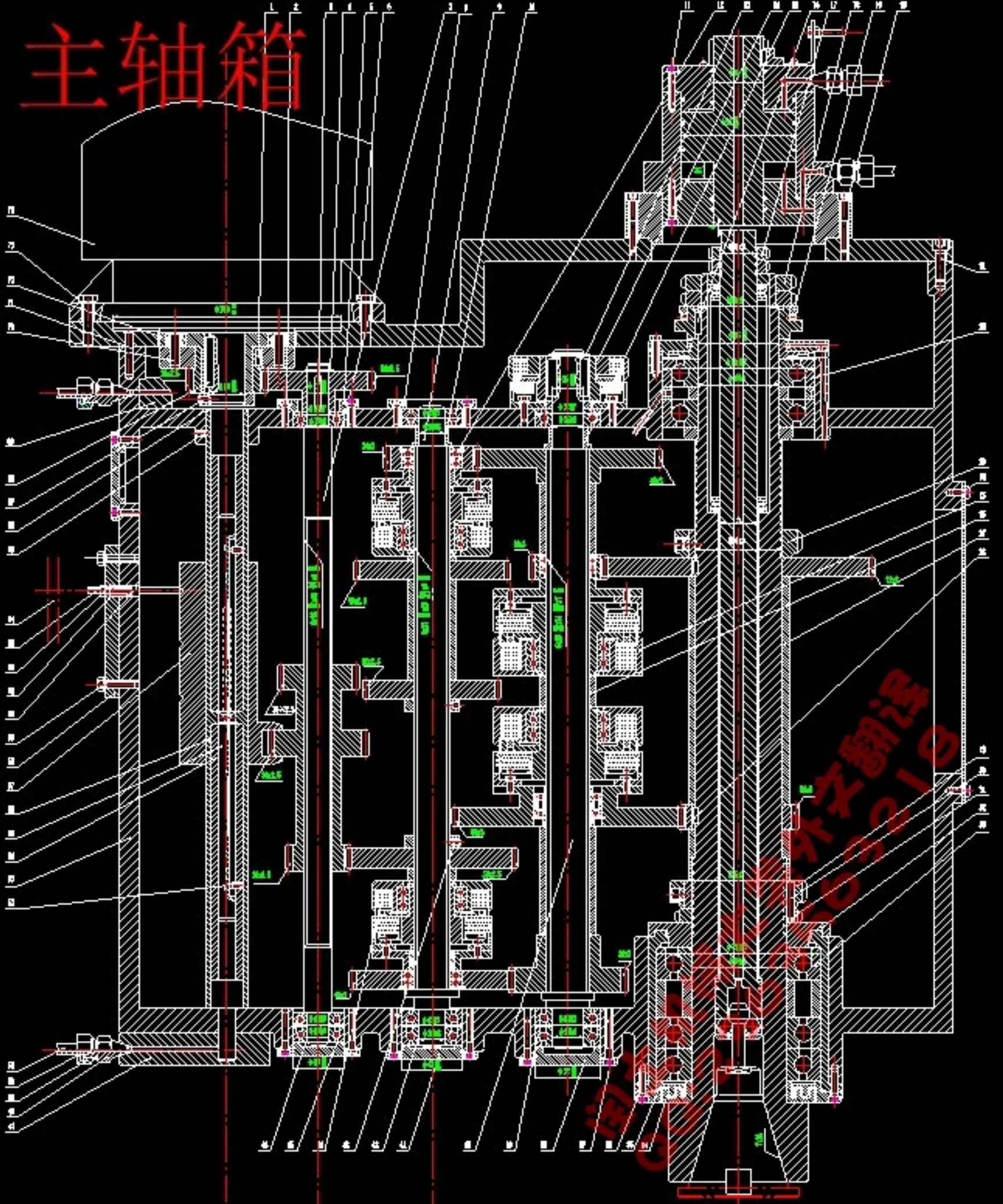
装配图
