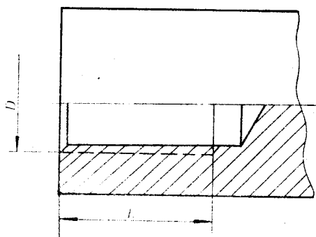
图1 内螺纹
