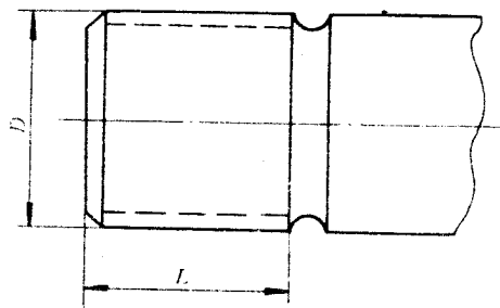
图3 外螺纹（无肩）
