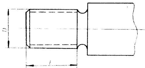
图2 外螺纹（带肩）
