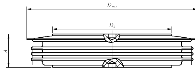
图2 外形尺寸
