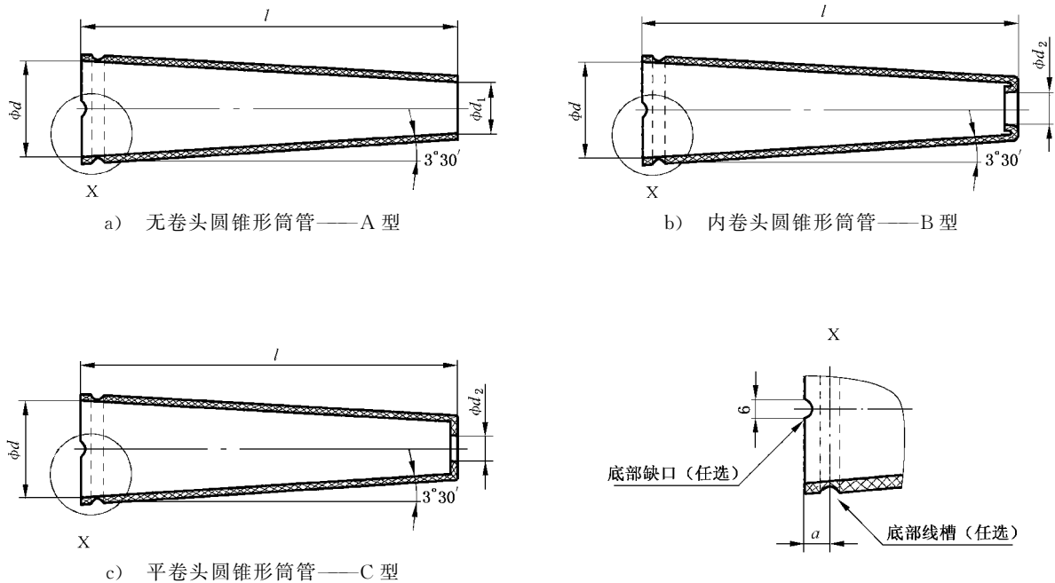
图 1 圆锥形筒管
