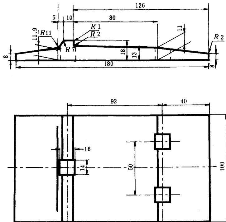
图 1 15kg/m 钢轨用垫板
