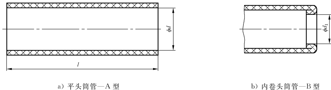
图 1 圆柱形筒管
