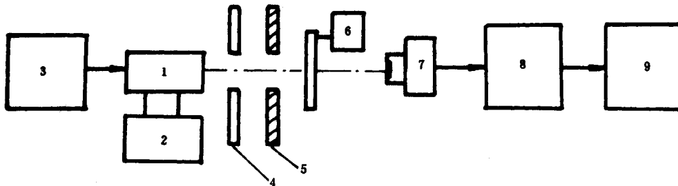
测量装置图
